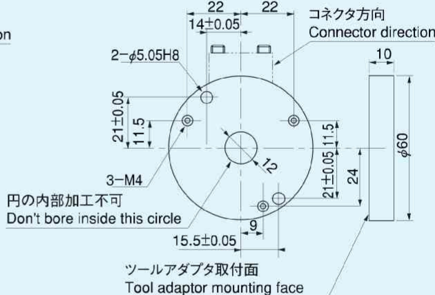
ツールアダプタプレート Tool adaptor plate
