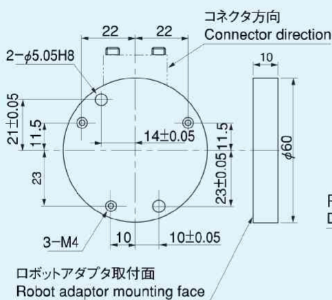
ロボットアダプタプレート Robot adaptor plate
