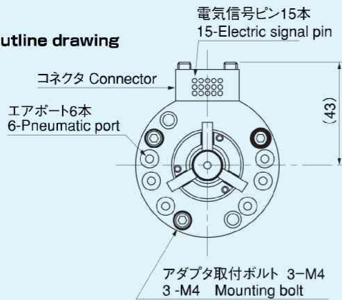
ロボットアダプタプレート Robot adaptor plate
